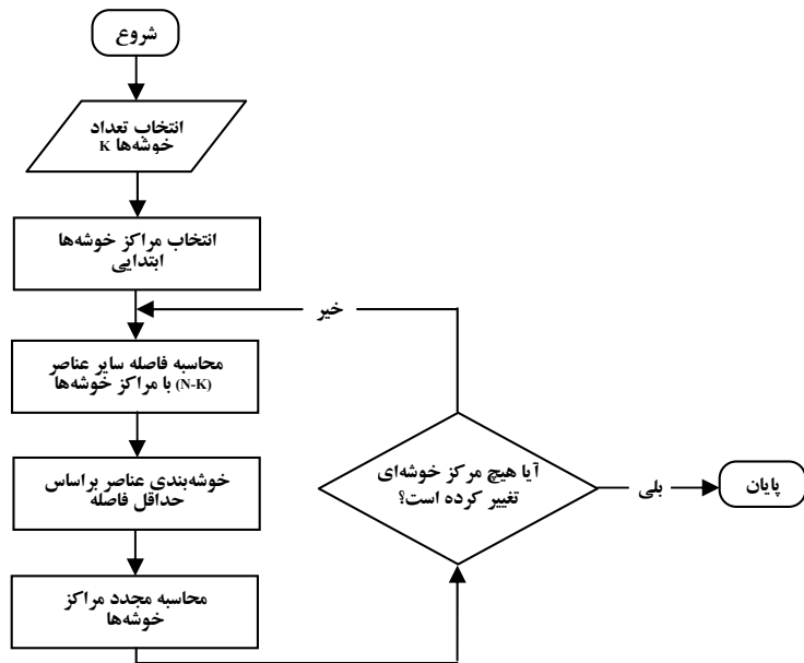
شکل ۲- الگوریتم Kmeans
